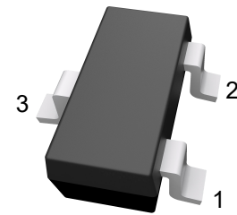
1.GND 2.VOUT 3.VIN
